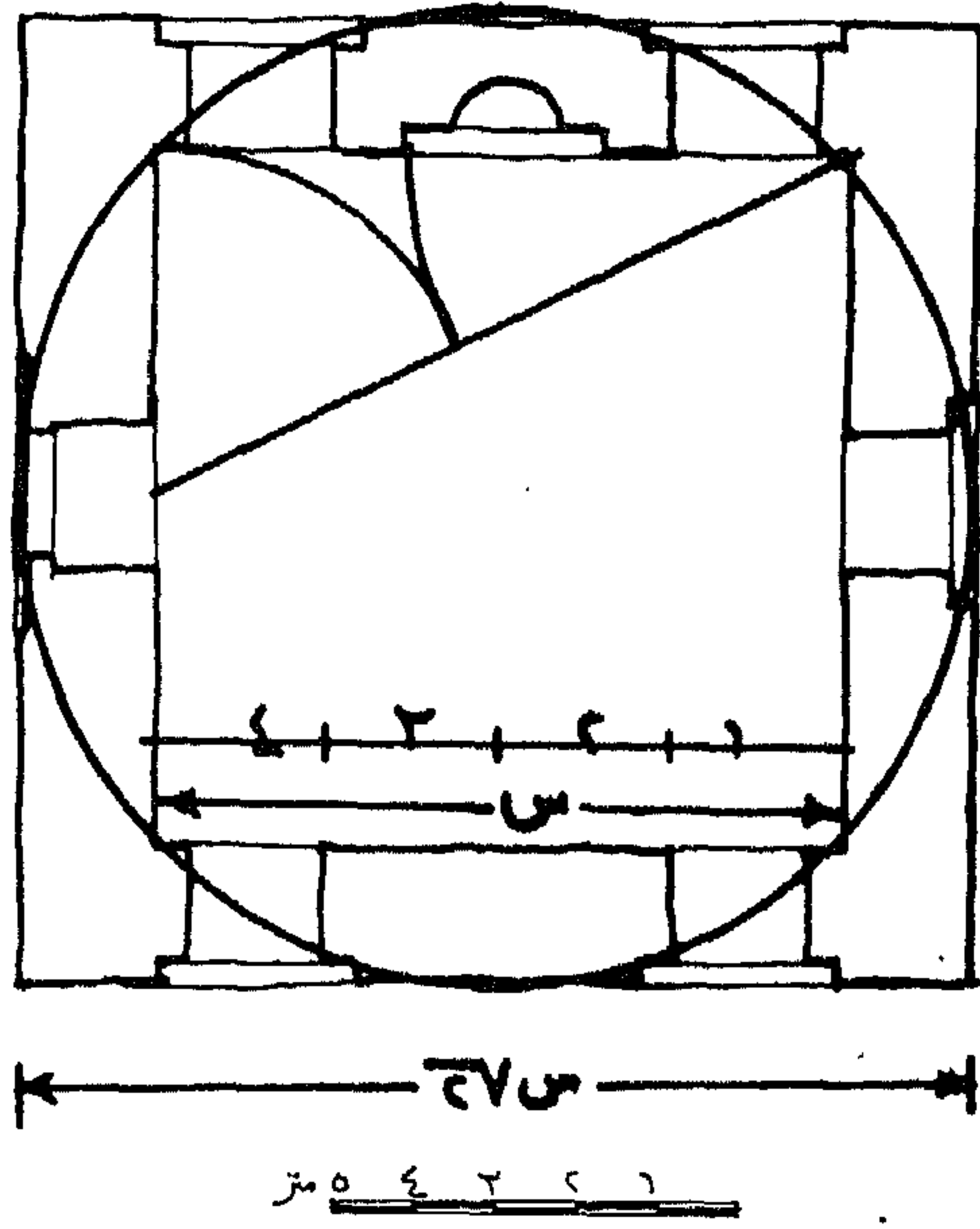
(١) قبة جانى بك الأشرفى . مسقط أفقى
