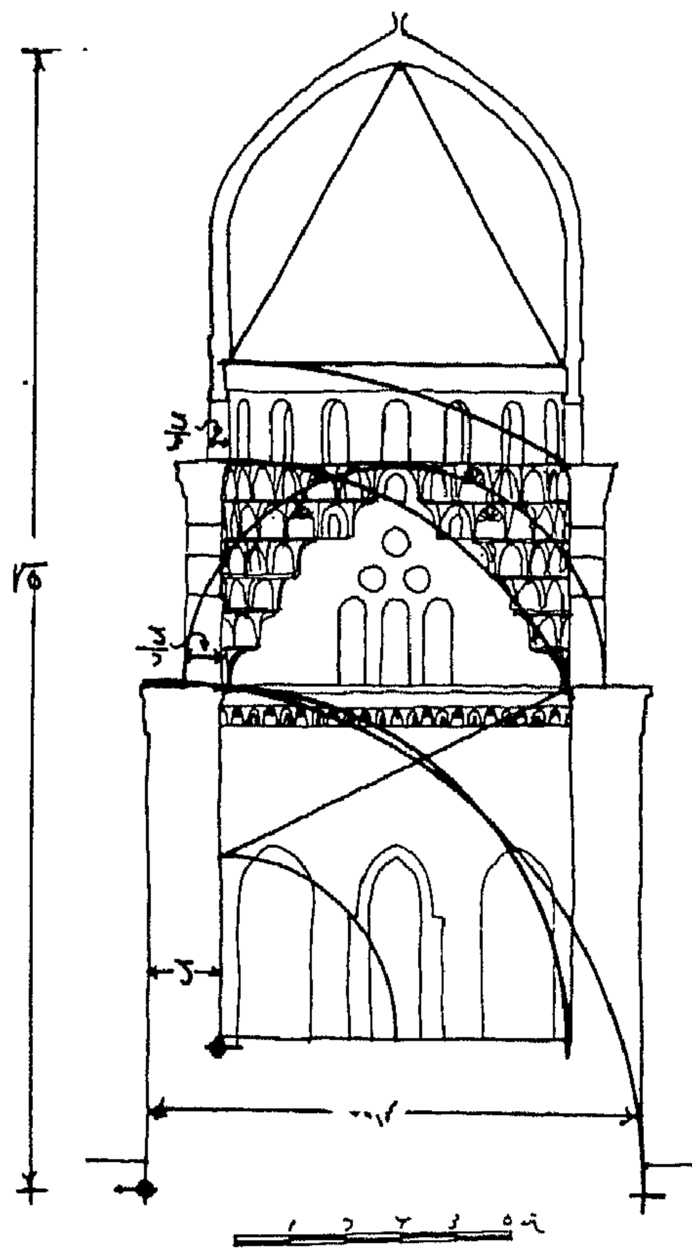
(٨) قبة السبع بنات . قطاع رأسى
