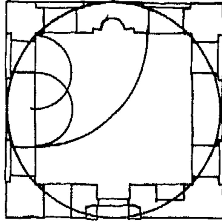
١٤٤٤ متر (٧) قبة السبع بنات . مسقط أفقى
