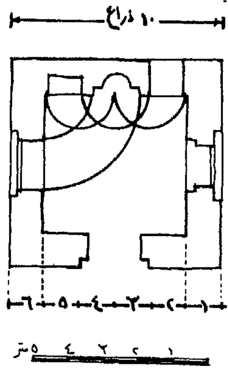
(٤) قبة نصر الله . مسقط أفقى
