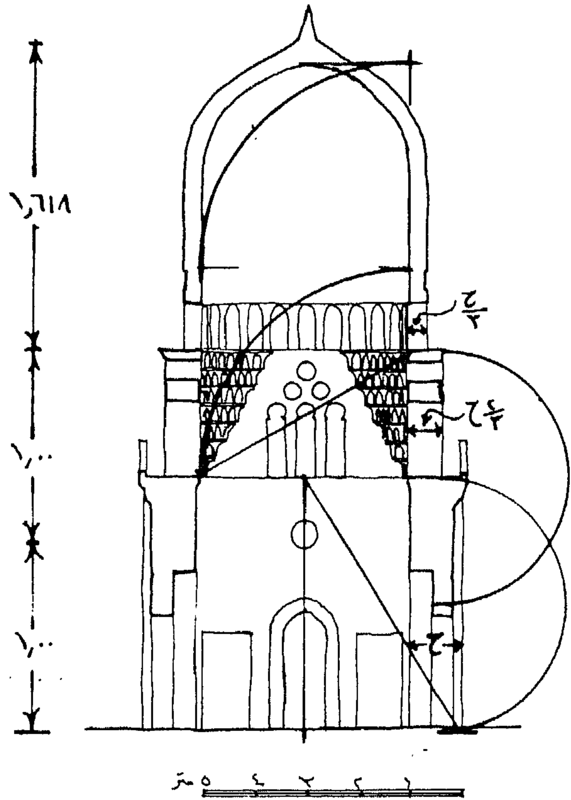
(٥) قبة نصر الله . قطاع رأسى
