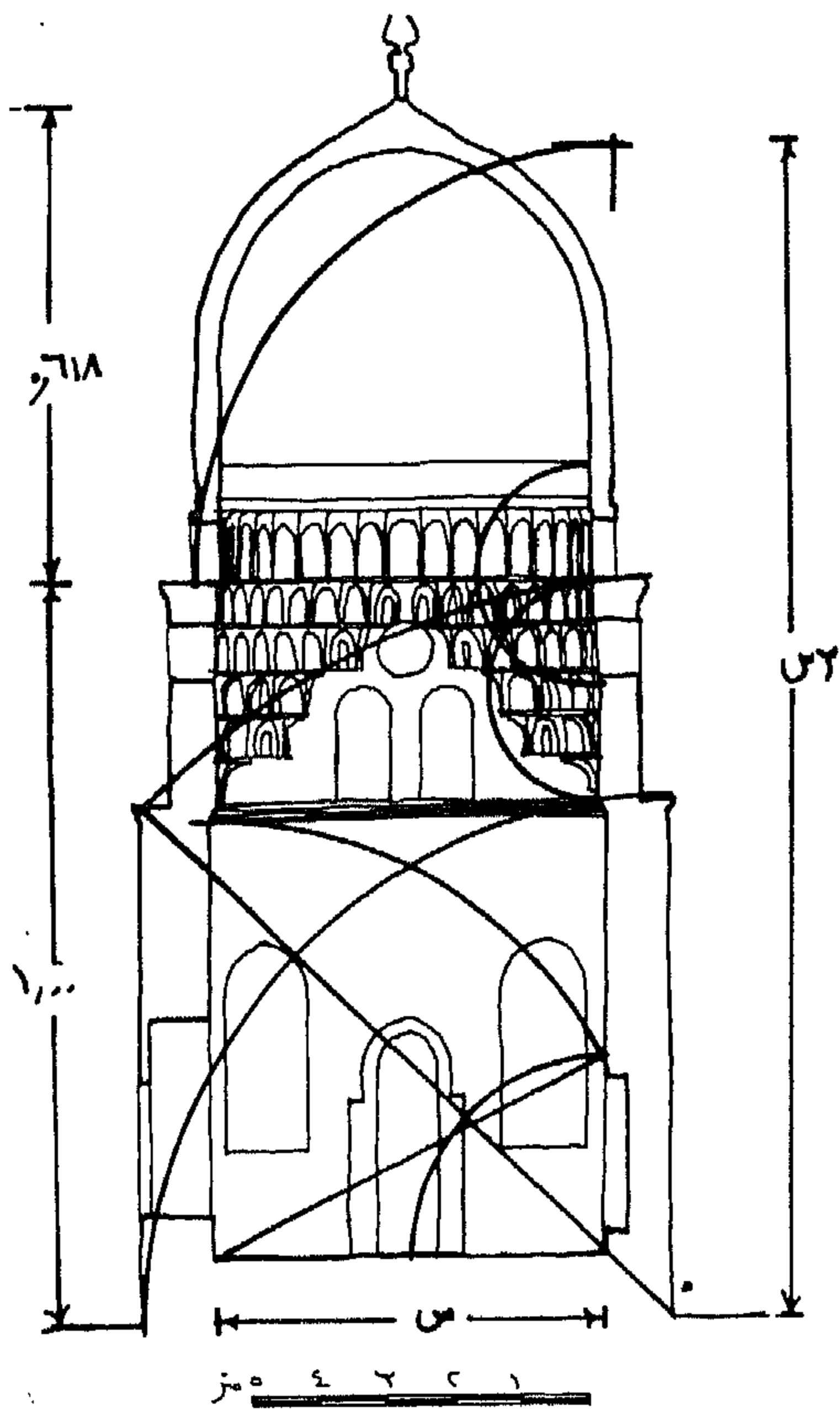
(٩) قبة برسبای البجاسى . قطاع رأسى
