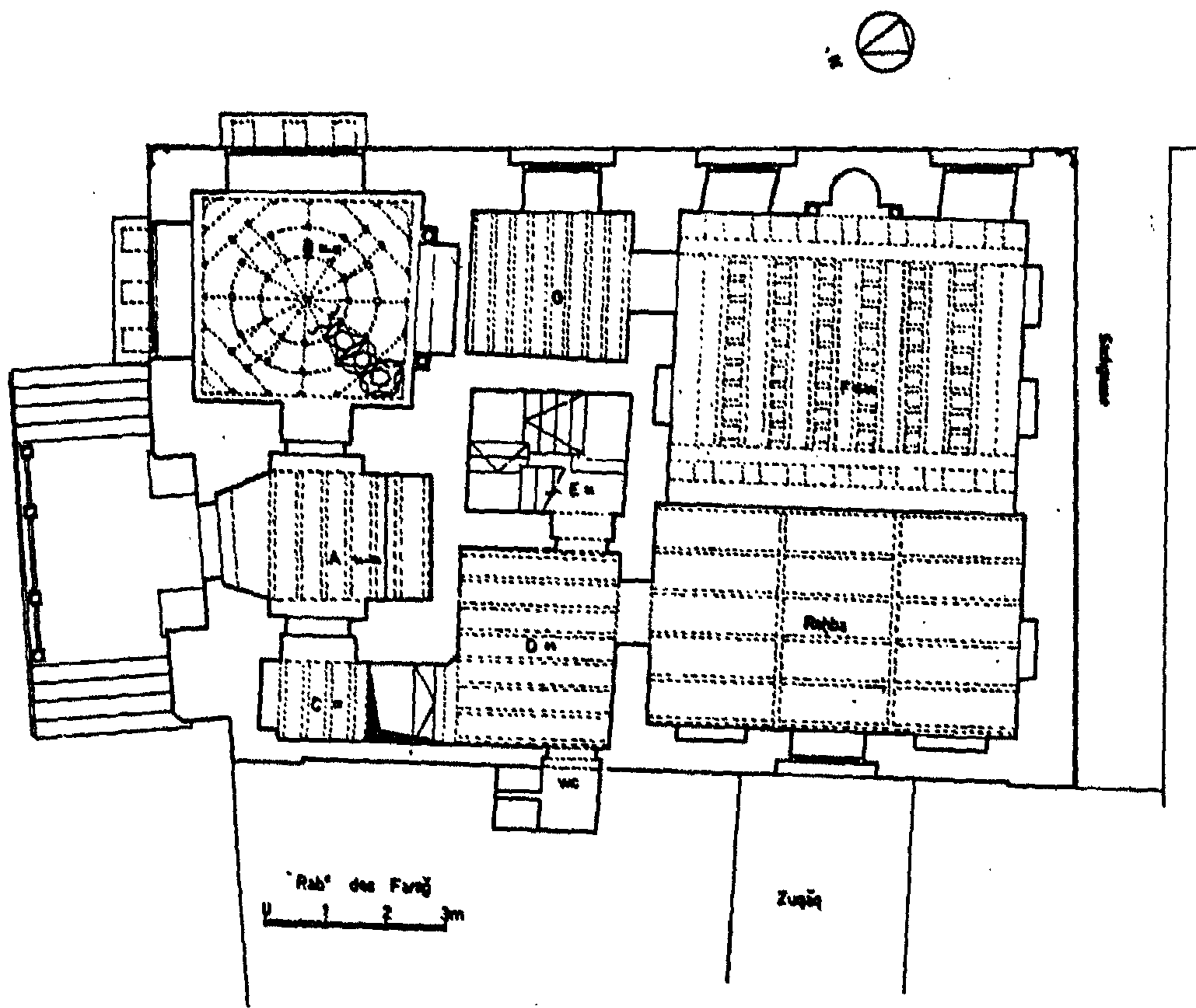
١- مسجد فرج بن برقوق - المسقط الأصلي (LAMEI)
