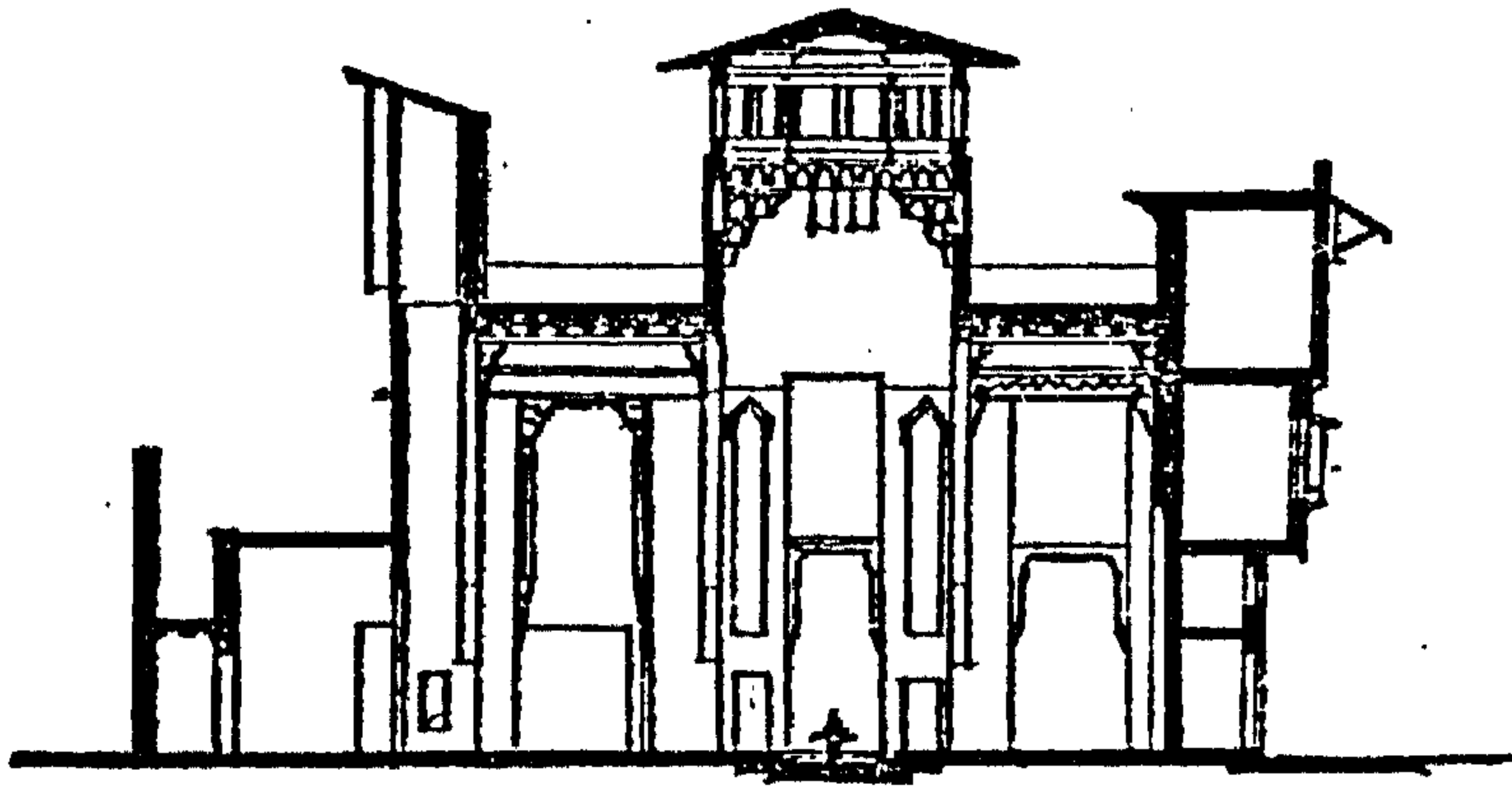
قطاع أ-أ قاعة عثمان كتحذا (عن د. كمال سامح)
