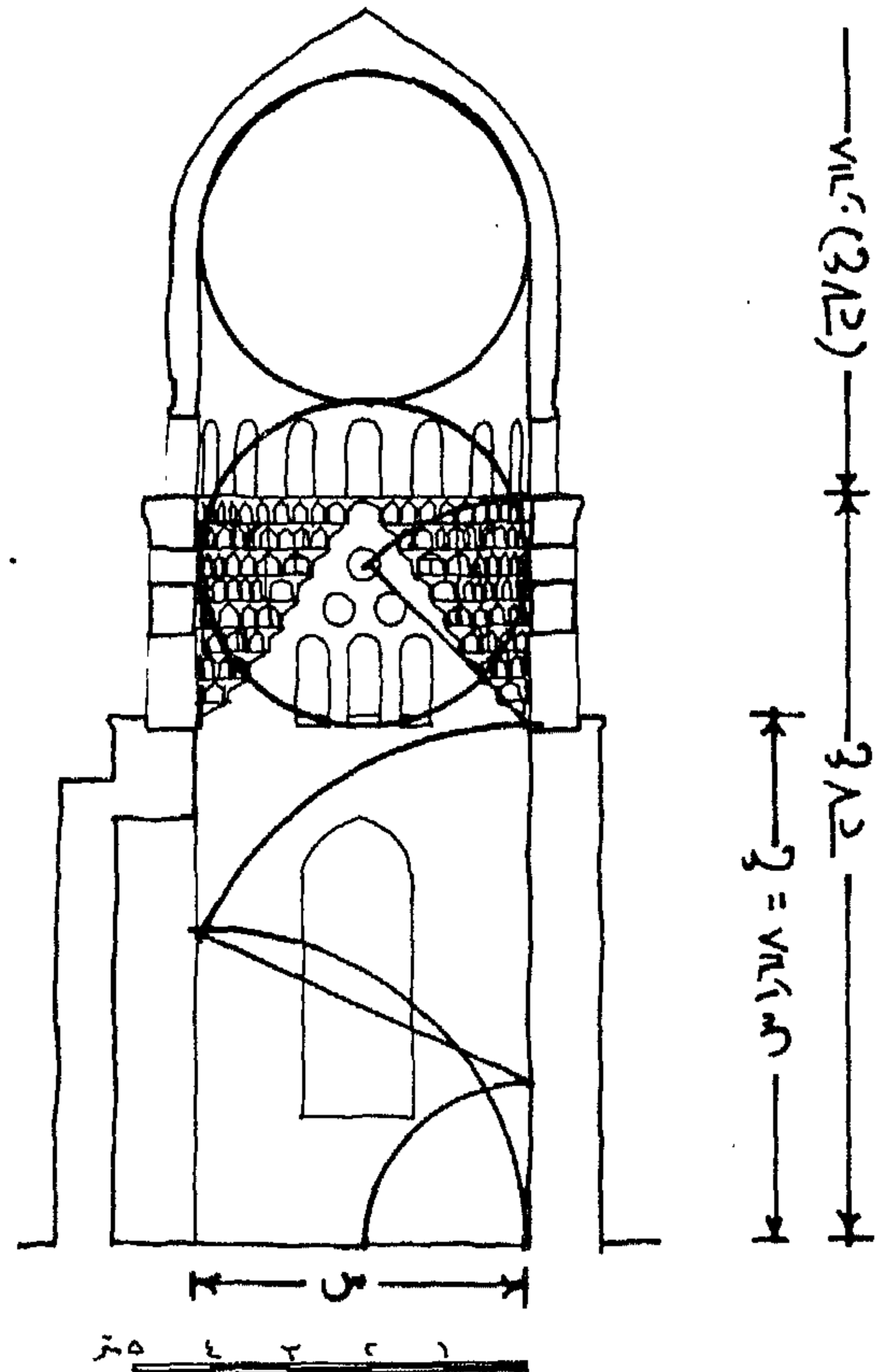
(١٣) قبة أزدمر . قطاع رأسى
