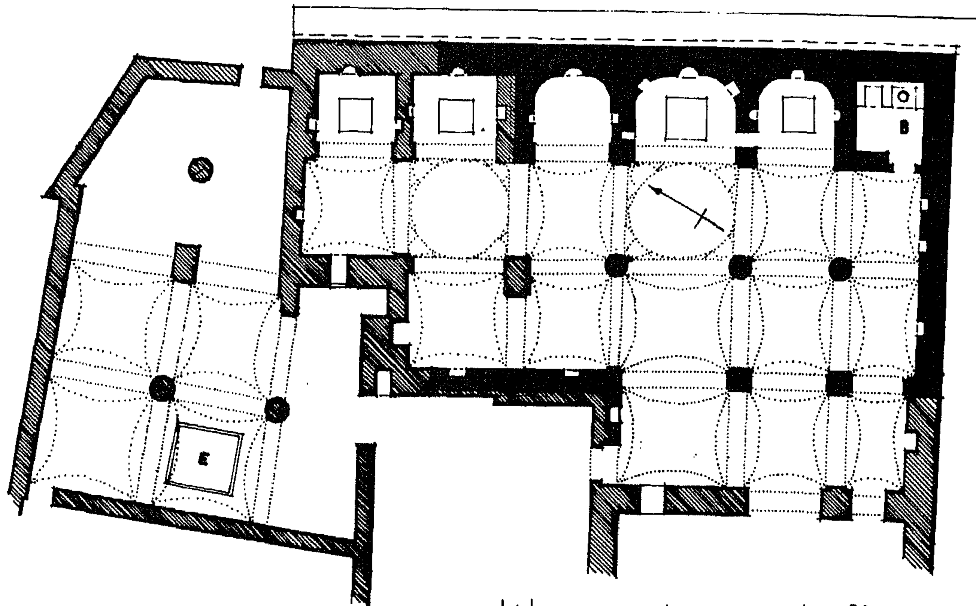
مخطط (٧) دير الملاك ميخائيل - نجع الدير شرق جرجا
