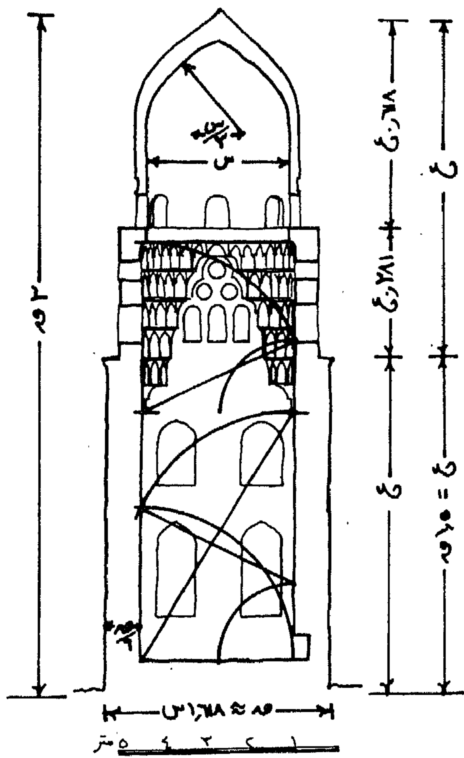
(11) قبة عصفور . قطاع رأسي
