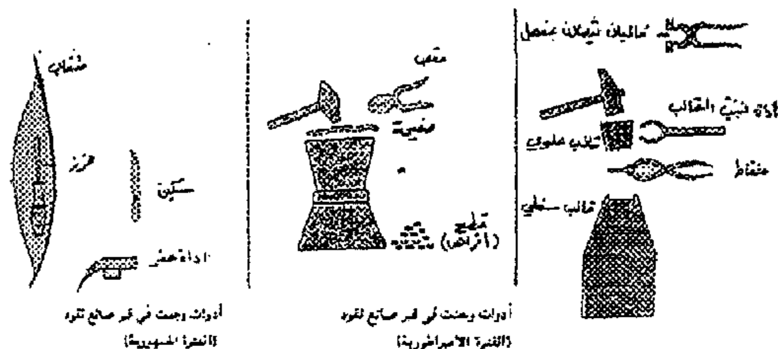
شكل ٧٢: رسوم لبعض الأدوات المستخدمة في عملية سك النقود في دار السك، توضح عملية إنتاج النقود في الفترة الرومانية. وقد استمر استخدام هذه الأدوات، وكذا الأساليب الفنية في دور السك بعد ذلك، القسوس: نميات نحاسية، ص ١٦٥ شكل ٤٥.
