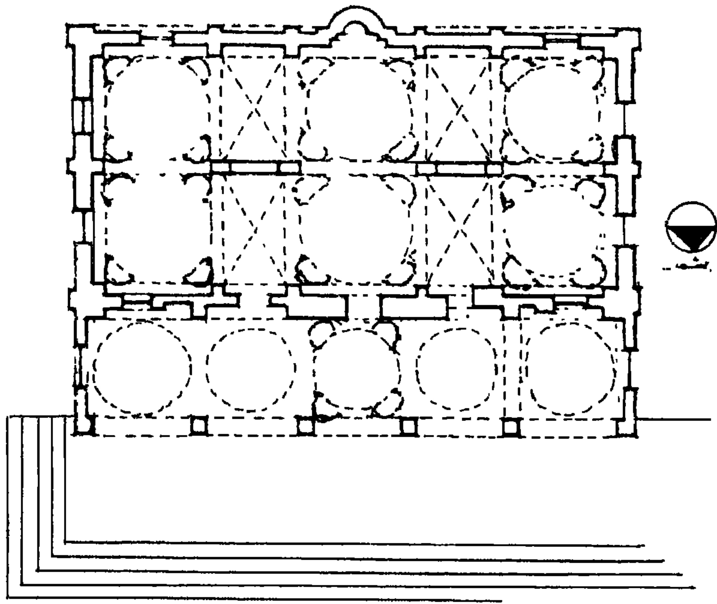
شكل ( ٤ ) : مسقط افقى لمسجد الغمامة بالمدينة المنورة .
