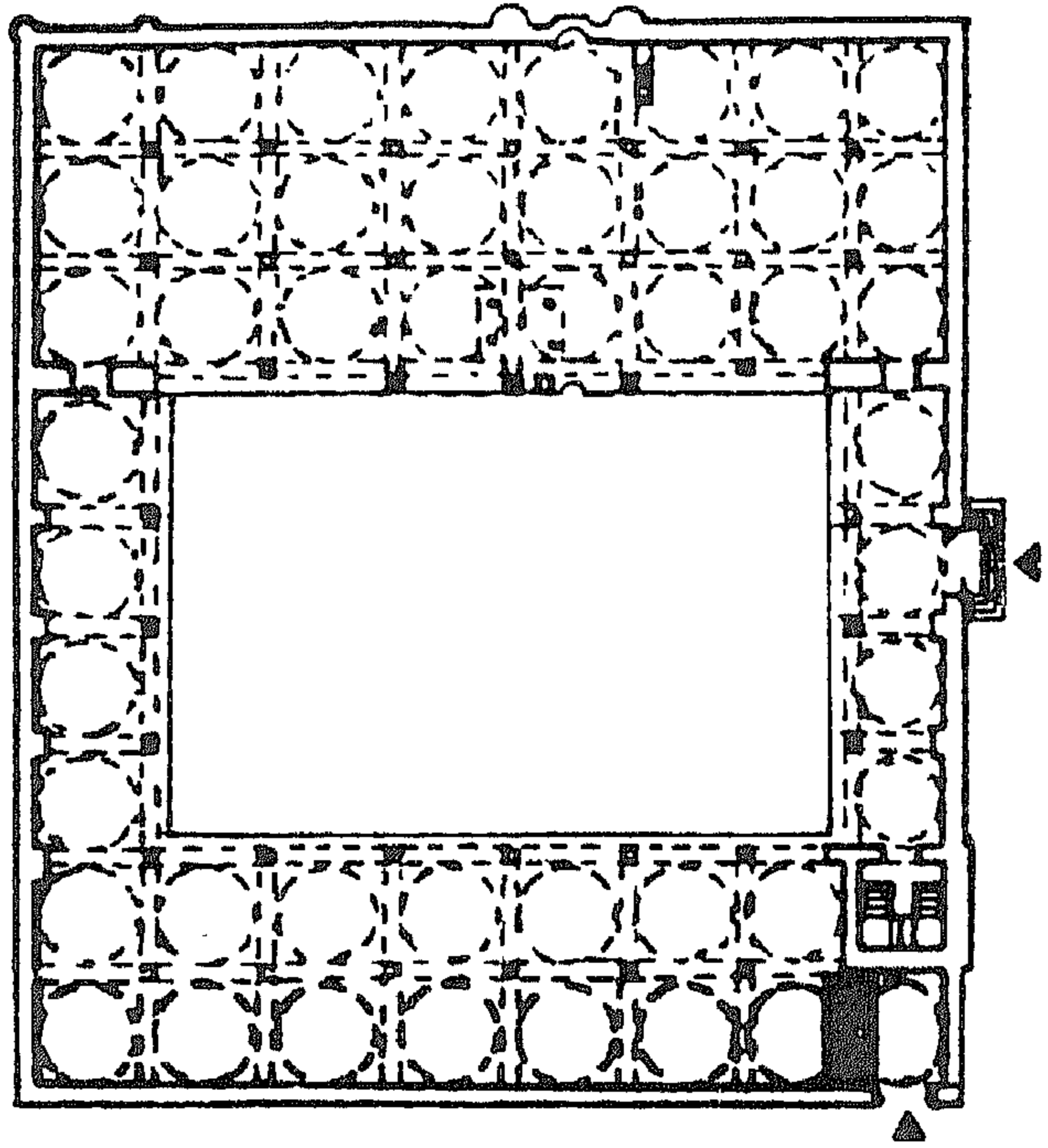
شكل ( ٥ ) : مسقط أفقى لمسجد قباء .
