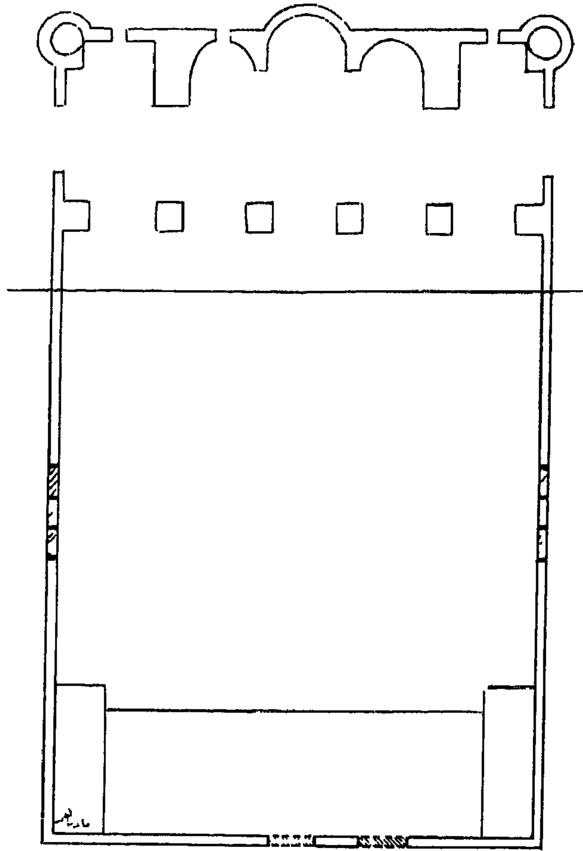
شكل رقم (١) تخطيط مسجد البعة الكبرى .
