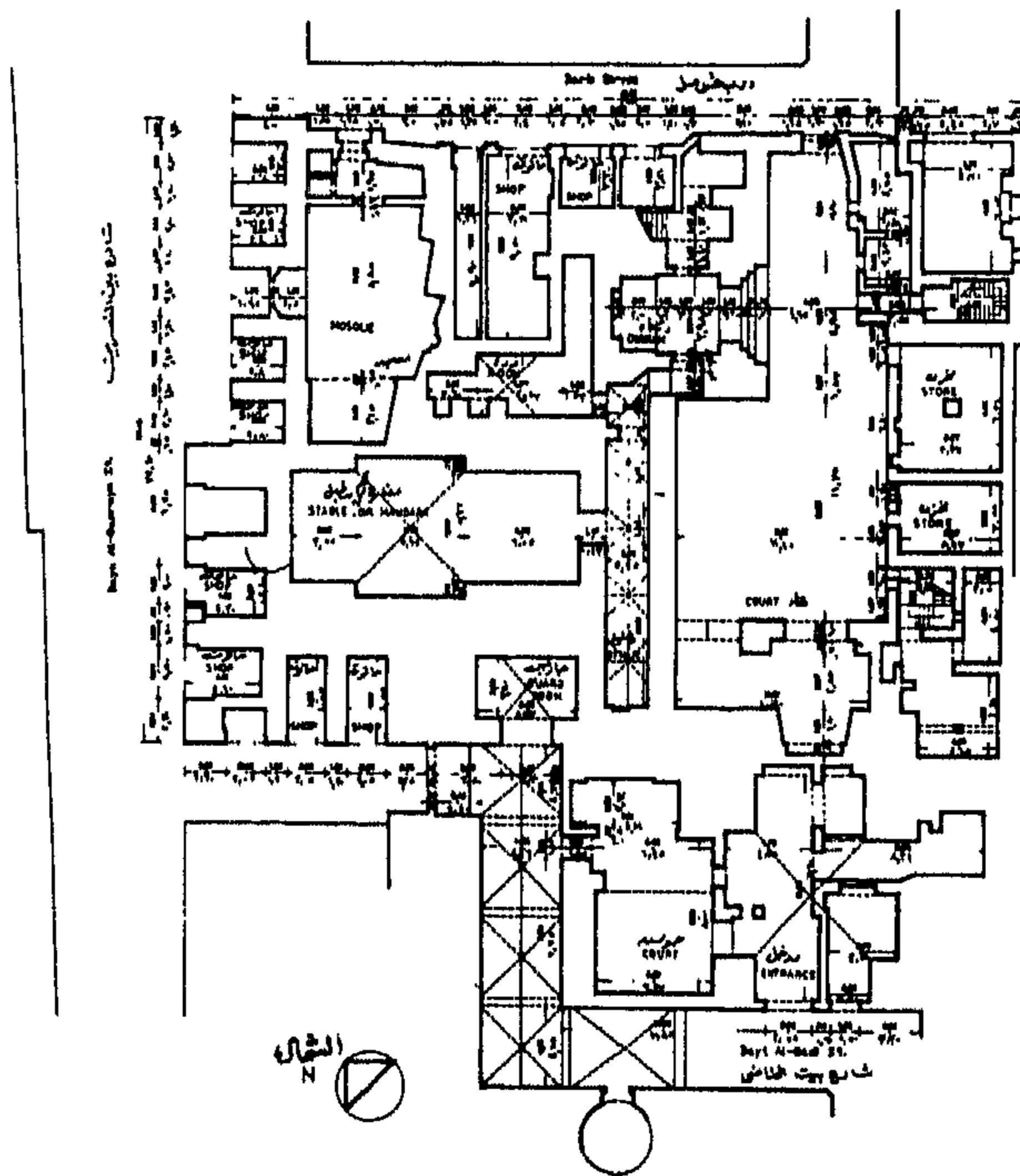
مسقط أفقى للدور الأرضى
