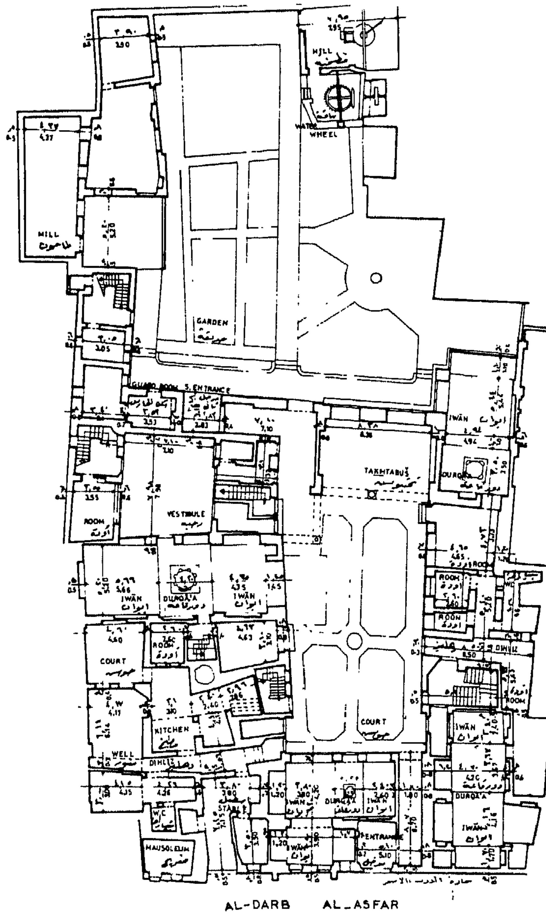
مسقط أفقى الدور الأرضى
