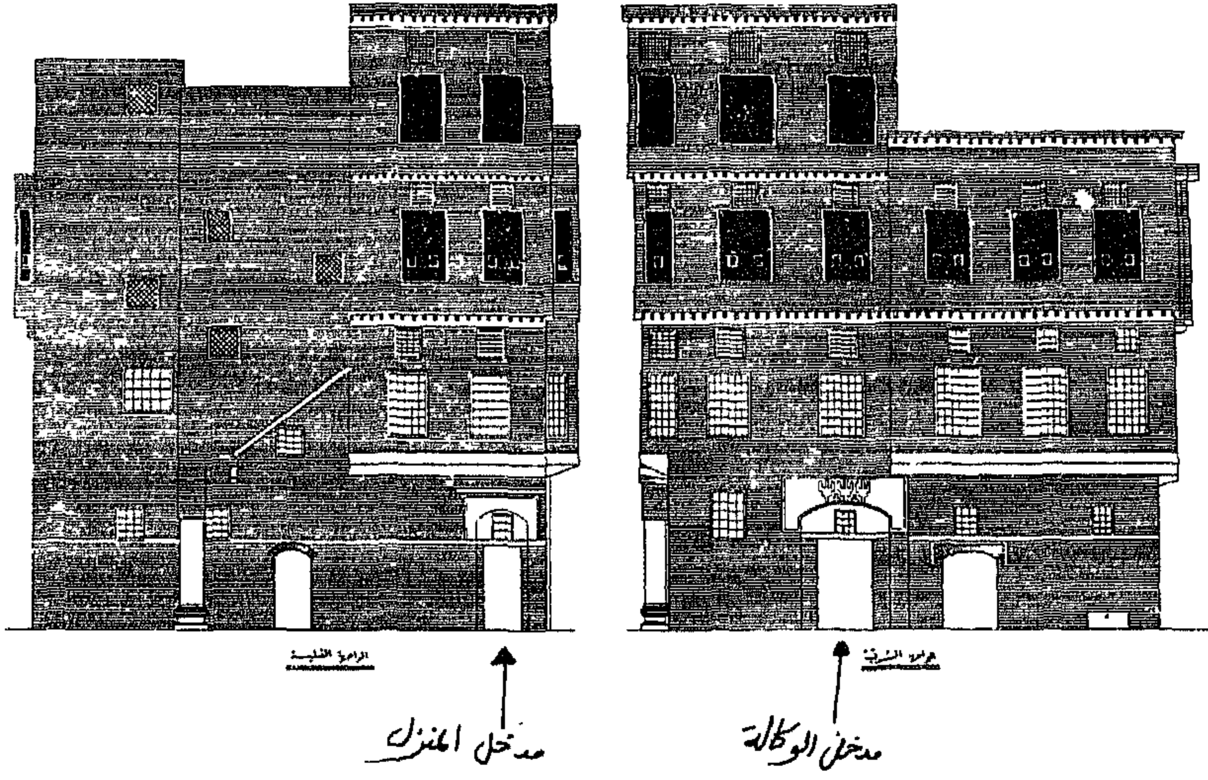
شكل رقم (٢٠) منزل عرب كركى الأثرى برشيد
