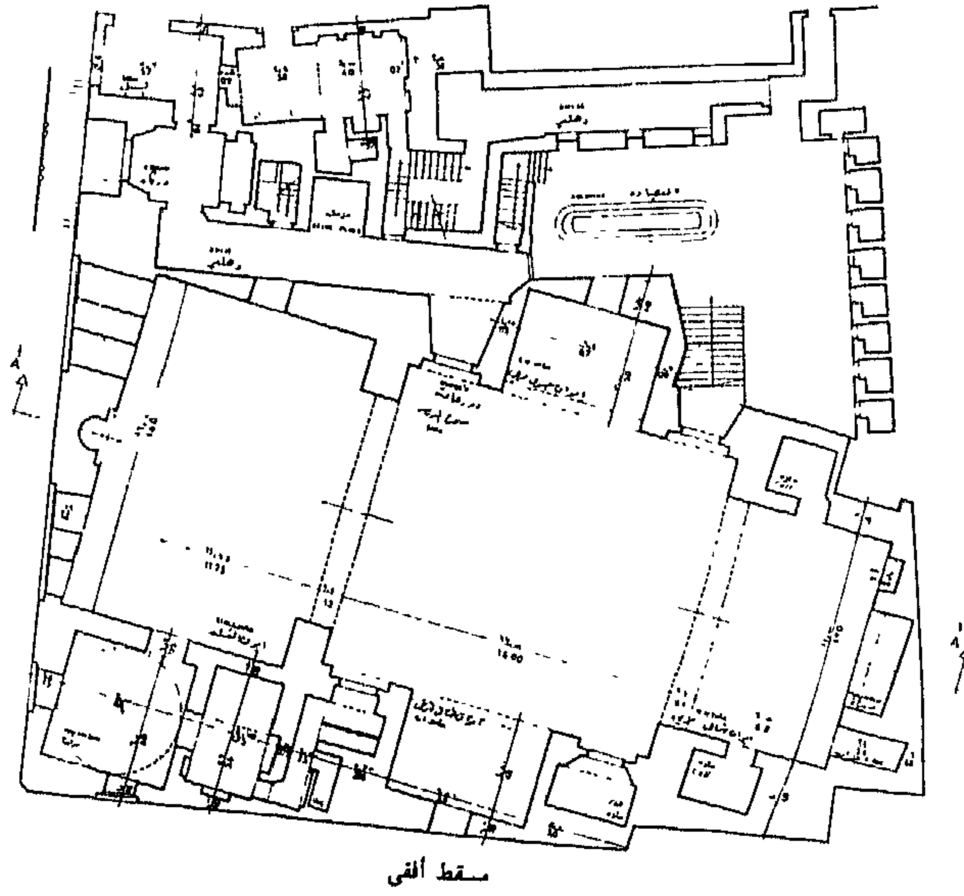
شكل رقم (٢) مسقط أفقي لمدرسة الأشرف برسباي
