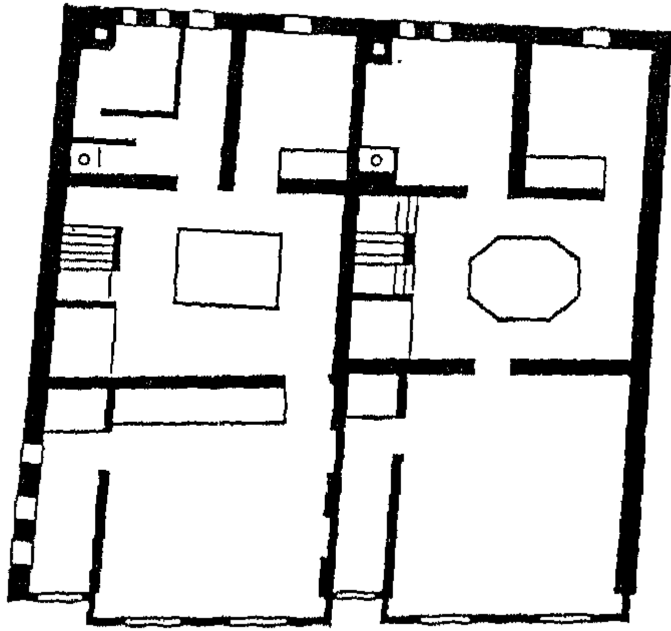
مسقط افقى الدور الثالث
