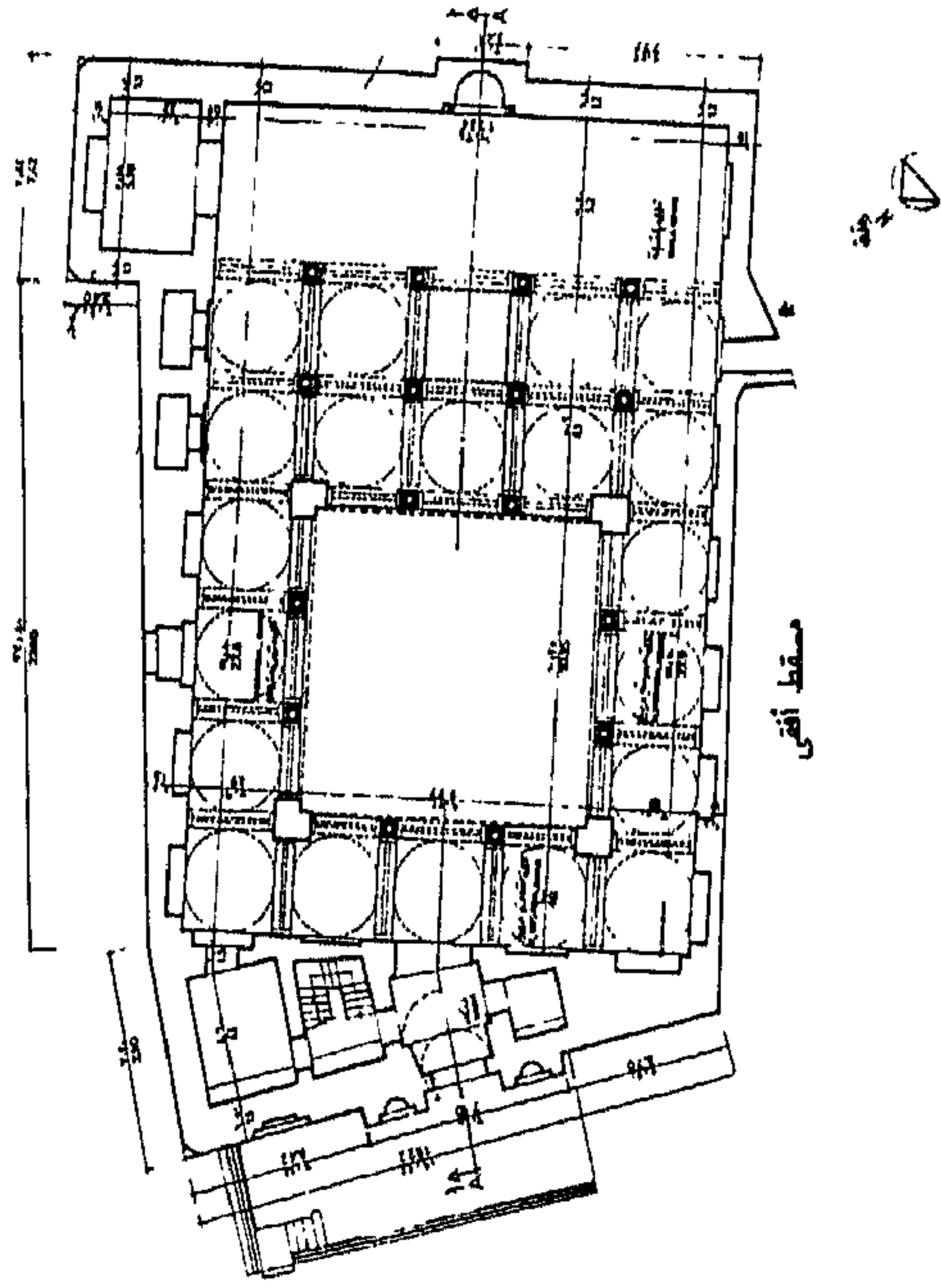
شكل رقم (١) مسقط أفقي لمسجد الأقرم
