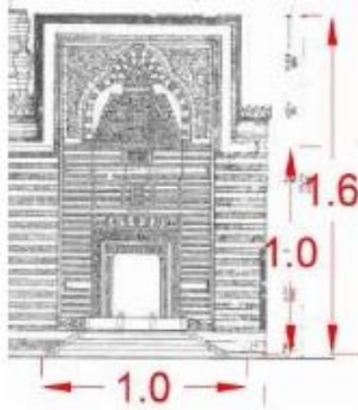
الشكل (2): يوضح نسب المدخل
