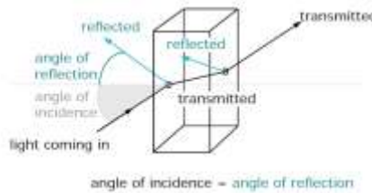
شكل (2) انعكاس ونفاذية وانكسار الضوء عند مروره مائلاً بزجاج شفاف
